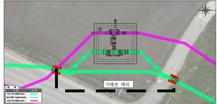
① 부단수 양단차단(SP, D800mm) 평면도 - 타이벨브실#1 (용수공급계획) 부단수차단장비 연결 후 장비와 장비간 가배관을 설치하여 용수공급 시행 (현장주소) 충남 서산시 성연면 명천리 63-1 일원
