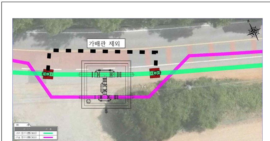
④ 무단수 양단차단(SP, D800mm) 평면도 - 타이벨브실#4 (용수공급계획) 무단수차단장비 연결 후 장비와 장비간 가배관을 설치하여 용수공급 시행 (현장주소) 충남 당진시 정미면 봉생리 347-8 일원
