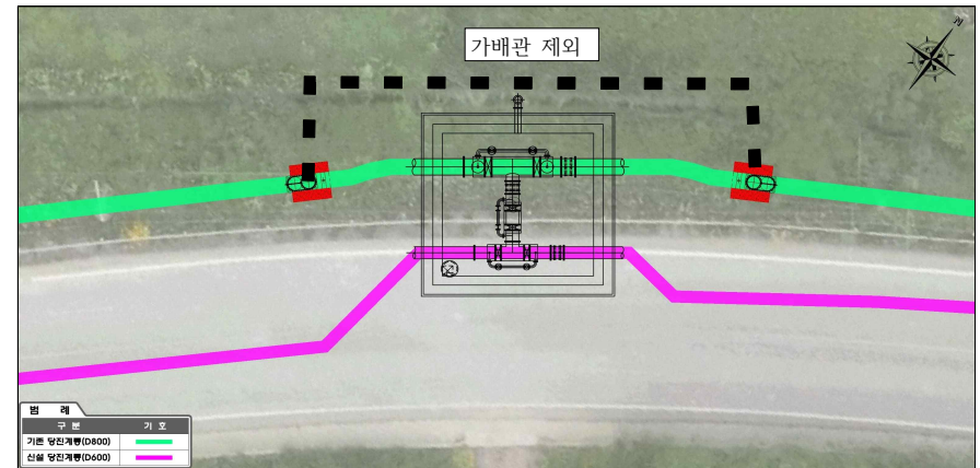
② 부단수 양단차단(SP, D800mm) 평면도 - 타이벨브실#2 (용수공급계획) 부단수차단장비 연결 후 장비와 장비간 가배관을 설치하여 용수공급 시행 (현장주소) 충남 당진시 정미면 우산리 265-1 일원
