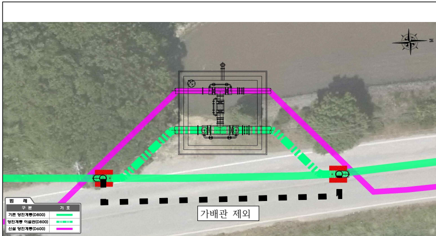
③ 무단수 양단차단(SP, D800mm) 평면도 - 타이벨브실#3 (용수공급계획) 무단수차단장비 연결 후 장비와 장비간 가배관을 설치하여 용수공급 시행 (현장주소) 충남 당진시 정미면 도산리 194-2 일원
